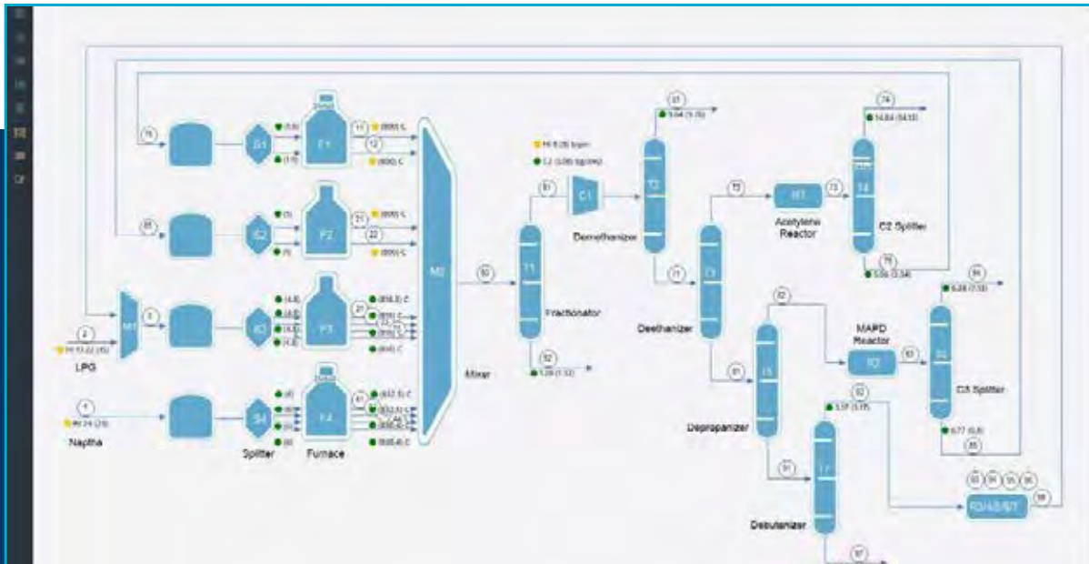
Tren de Olefinas de Aspen GDOT
